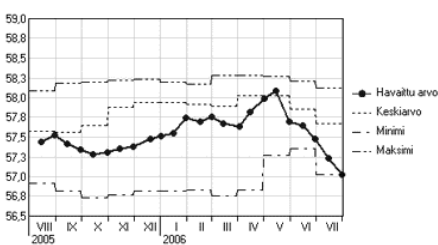
Pohjavedenkorkeus - Groundwater level 0=N60 + 0.00M
