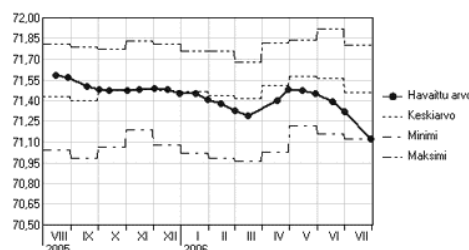
Pohjavedenkorkeus - Groundwater level 0=N60 + 0.00M
