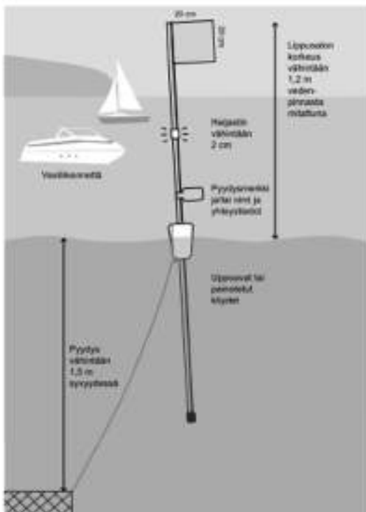
Kuva 1. Vesiliikenteen käyttämillä alueilla pyydys on merkittävä 1,2 metriä vedenpinnan yläpuolelle ulottuvaan salkoon kiinnitetyllä vähintään 20 senttimetriä leveällä ja korkealla neljän muotoisella lipulla. (Pirros Anu Väitalo/KKL)
